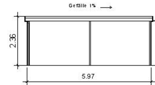
LÄNGSSCHNITT
